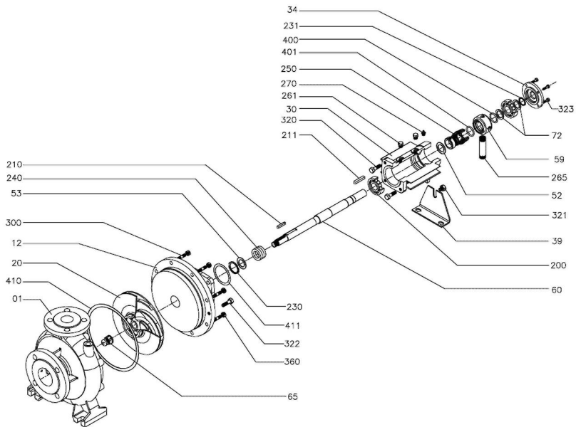
Рисунок 14: В РАЗОБРАННОМ ВИДЕ
