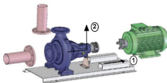
Рисунок 10: Демонтаж - 3
