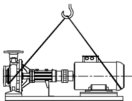
Рисунок 2: Транспортировка насосной группы
