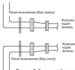
Рисунок 5: Система трубопроводов
