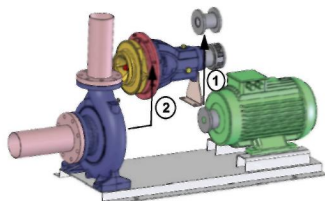
Рисунок 9: Демонтаж - 2
